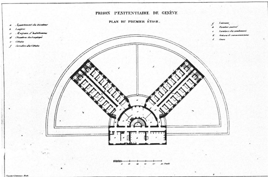
Figure 14: Tour Maitresse prison, Geneva, architect Samuel Vaucher-Crémieux, 1825: plan (Roth, Pratiques Pénitentiaires et Théorie Sociale , plate 4 following p.290)
